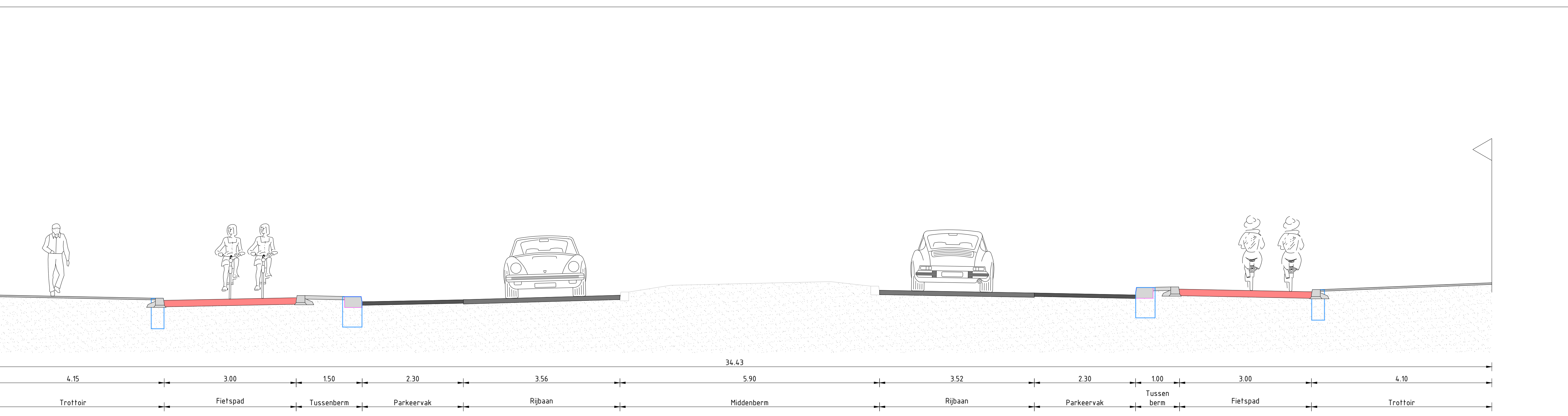
Dwarsprofiel F-F Schaal 1:50
