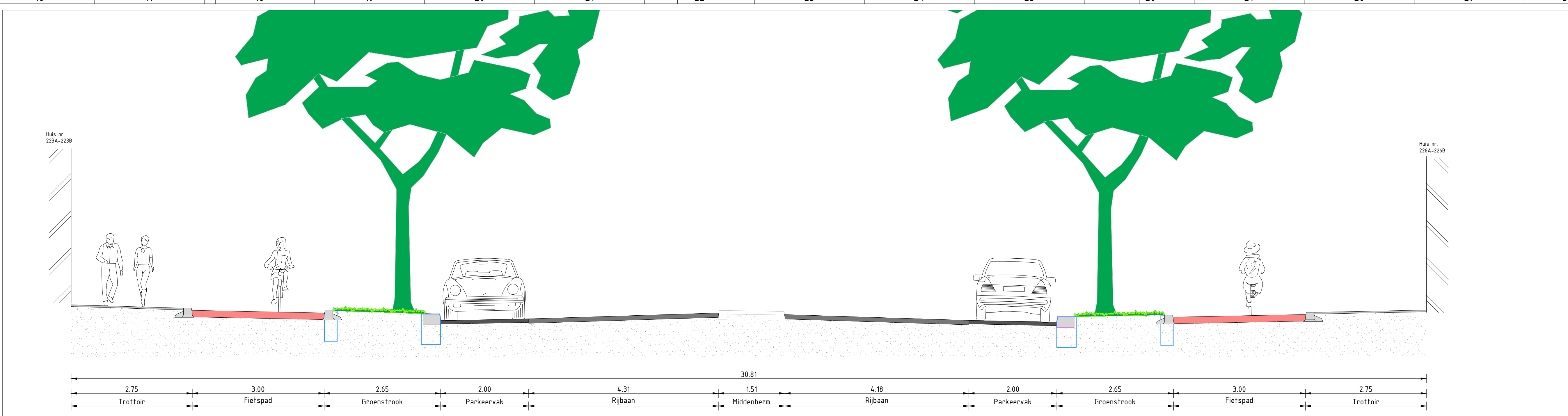
Dwarsprofiel B-B Schaal 1:50
