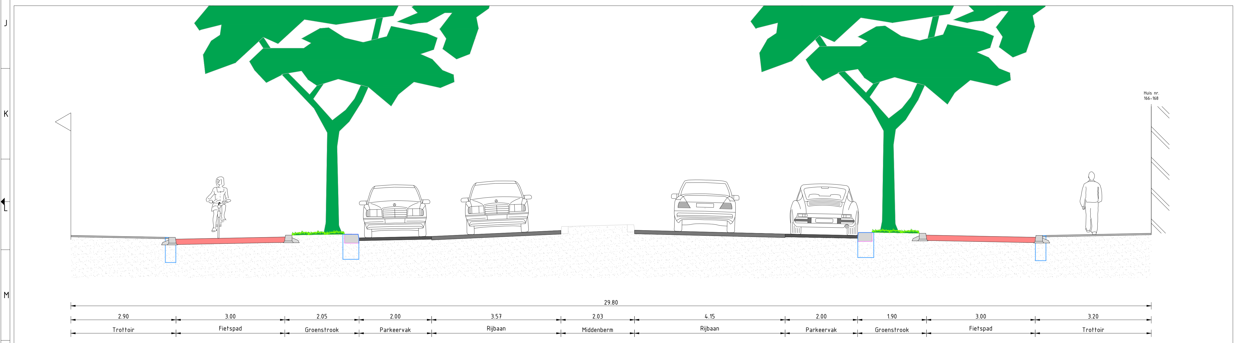
Dwarsprofiel E-E Schaal 1:50
