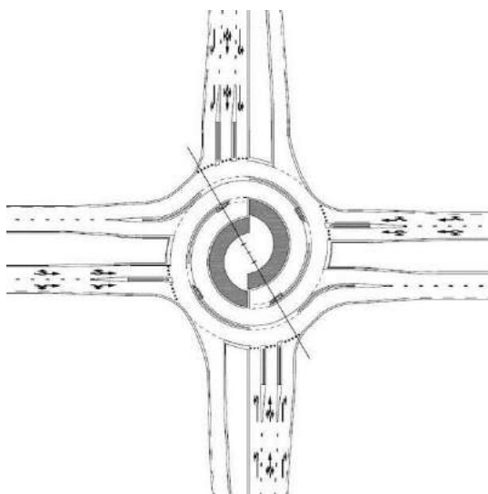
Figuur 7: Spiraalrotonde
