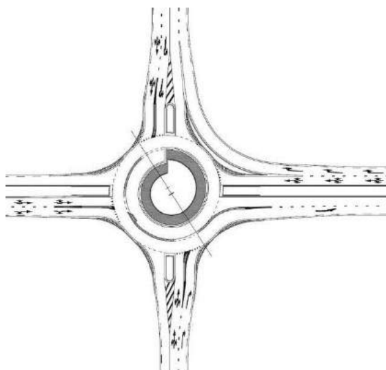
Figuur 8: Knierotonde
